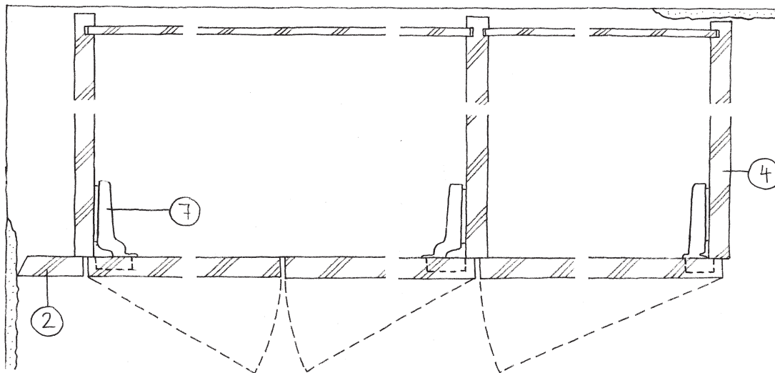
Pianta
