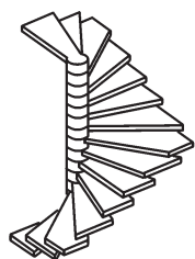
escalier en colimaçon à marches ouvertes plan rectangulaire
